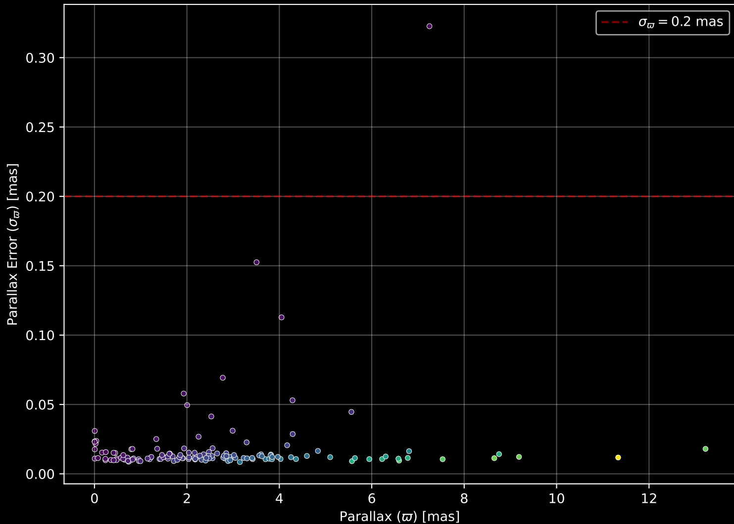
APOGEE DR17 Field: [282-37-O_TESS] Parallax Quality (n= 140)
