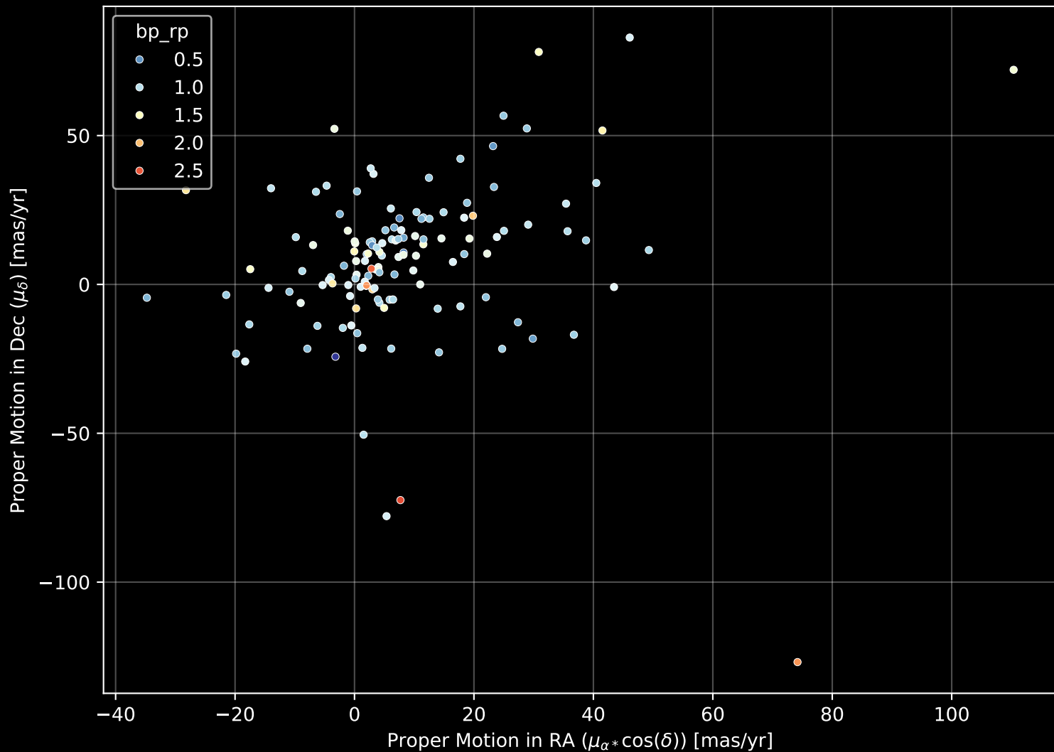
APOGEE DR17 Field: [282-37-O_TESS] Proper Motion Diagram (n= 140)
