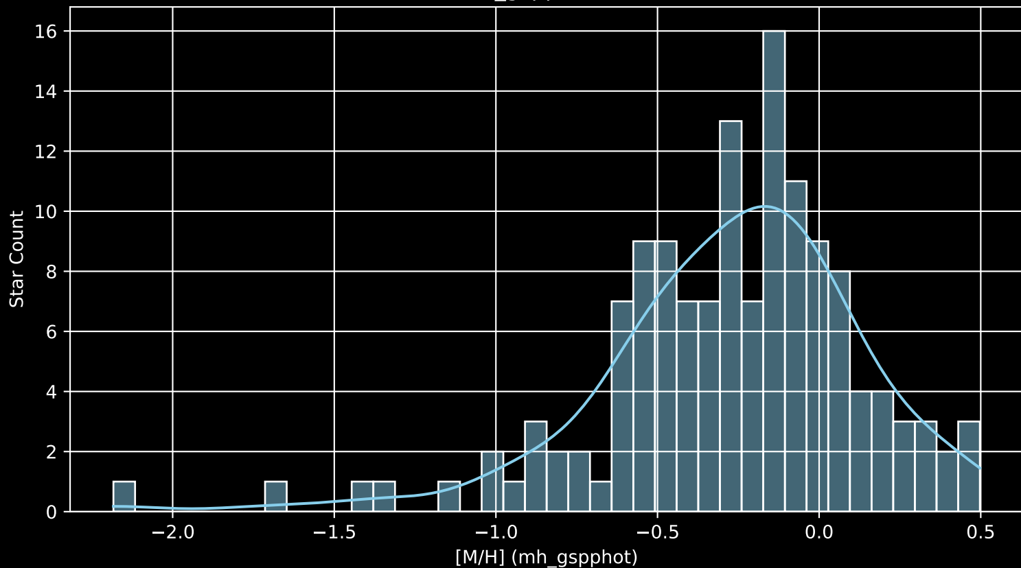
APOGEE DR17 Field: [282-37-O_TESS [M/H] (mh_gspphot) (n= 138)
