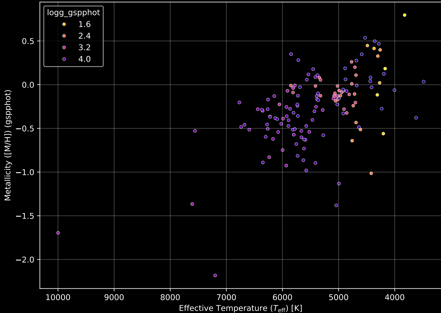
APOGEE DR17 Field: [282-37-O_TESS] Stellar Population Parameters (n= 140)
